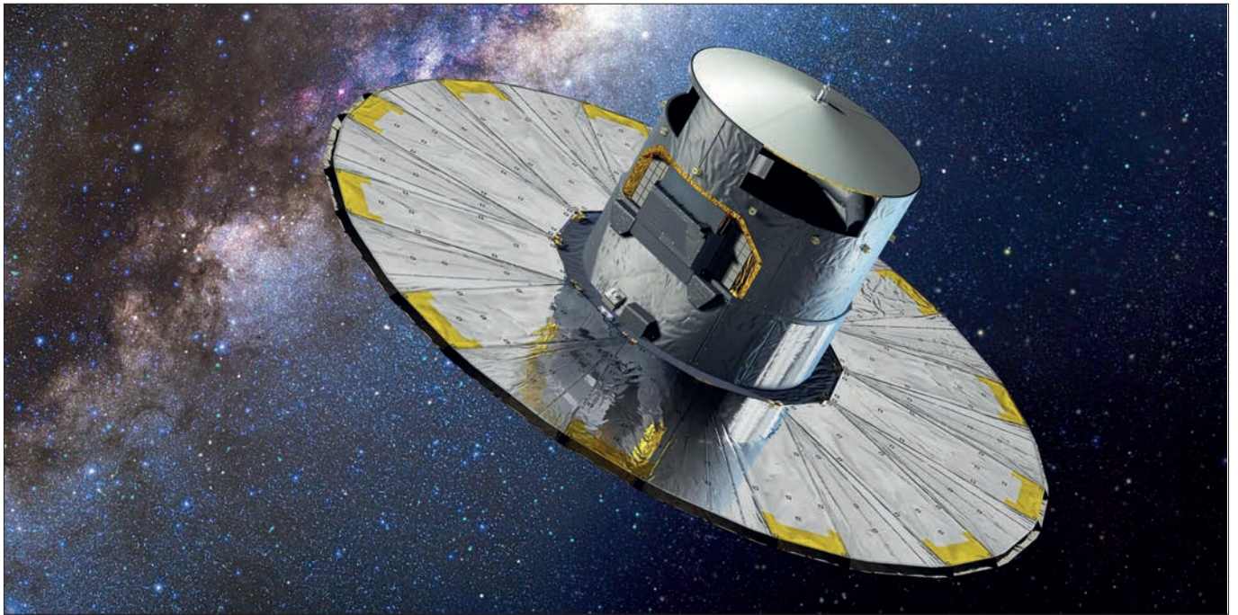
El telescopi espacial Gaia va ser col·locat a l'espai l'any 2013.
