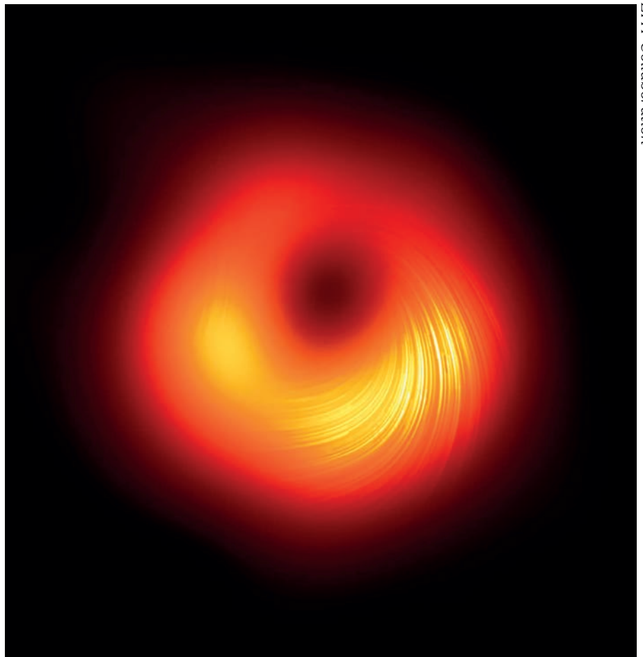
EHT Collaboration
