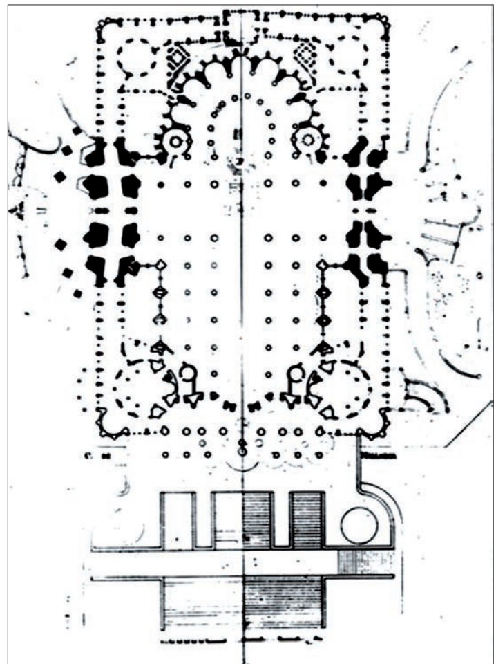
Plano de urbanización elaborado por Gaudí.
