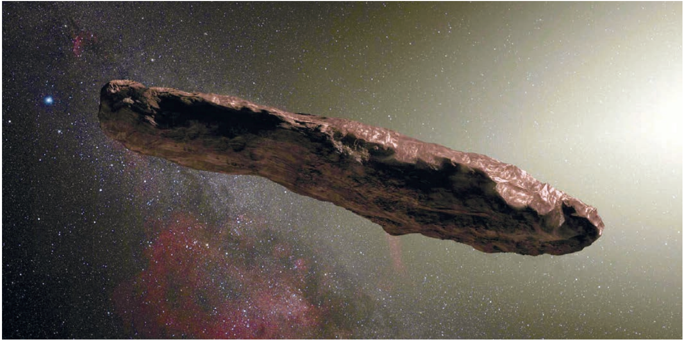
Recreación artística del objeto interestelar 'Oumuamua. / M. Kornmesser / ESO
