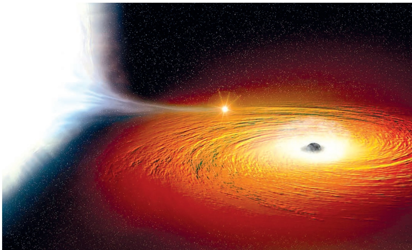
Recreación de un agujero negro supermasivo.
