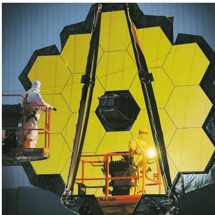
Ingenieros realizando una inspección de luz blanca al Telescopio James Webb de la NASA en la sala limpia del Centro Goddard de Vuelos Espaciales (NASA/Chris Gunn).
