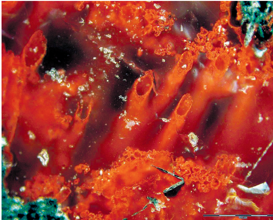
Tubos de hematites de la ventilación hidrotermal que se pueden haber formado por las bacterias oxidadoras de hierro que hipotéticamente se desarrollaron en el NSB (siglas en inglés de Citurón Supracortical de Nuvvuagittuq) y que podrían ser los restos de algunas de las primeras formas de vida en la Tierra.
