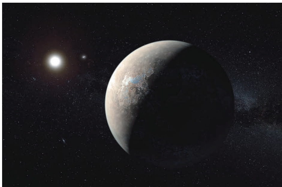
Impresión artística de «Proxima Centauri».
