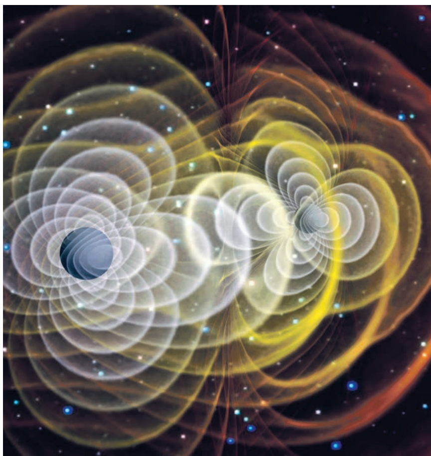
Simulación realizada por ordenador de ondas gravitacionales producidas por dos agujeros negros en órbita (imagen: NASA).
