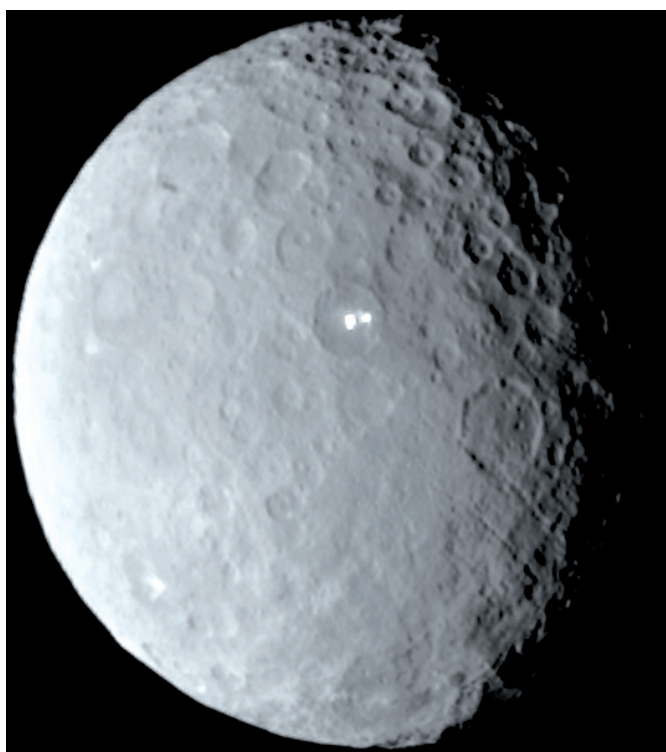
Ceres. Foto enviada per la sonda «Dawn» on es poden apreciar les taques brillants que la NASA troba tan interessants.
