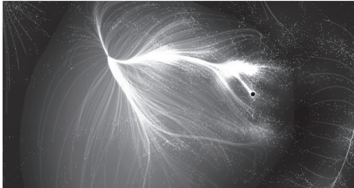
Supercúmulo «Laniakea», el punt més negre representa la ubicació de la Via Làctia. (Fotograma del vídeo d'una simulació per ordinador de la revista «Nature»)
