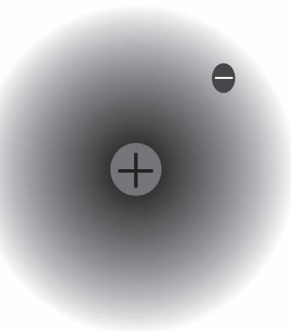
Átomo del hidrógeno, con un protón y un electrón.
