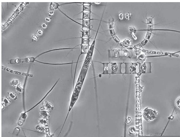
Vista al microscopio de células diatomeas marinas (« Rhizosolenia setigera »), importante grupo de fitoplancton.
