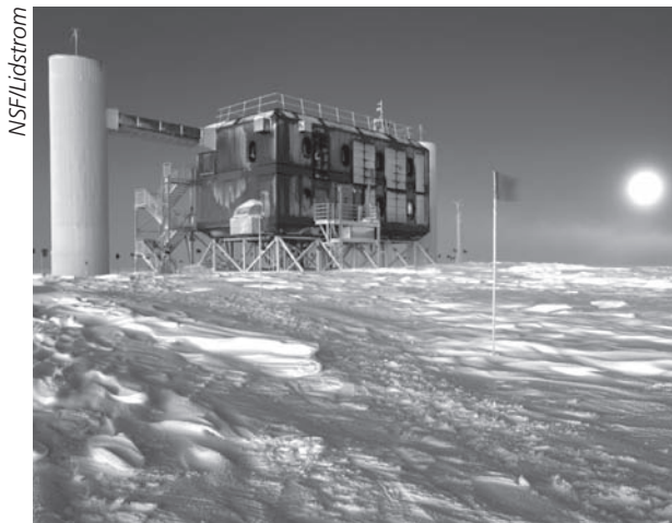
Laboratori del «IceCube» a l'Antàrtida.
