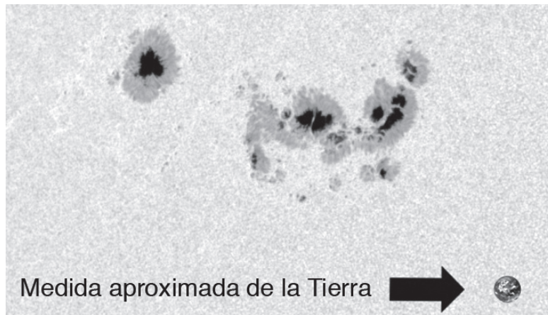
Mancha solar AR 1654, el 13 de enero, y tamaño de la Tierra en comparación a ella.
