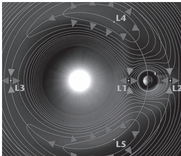
Los cinco puntos de Lagrange del sistema Sol-Tierra (NASA).
