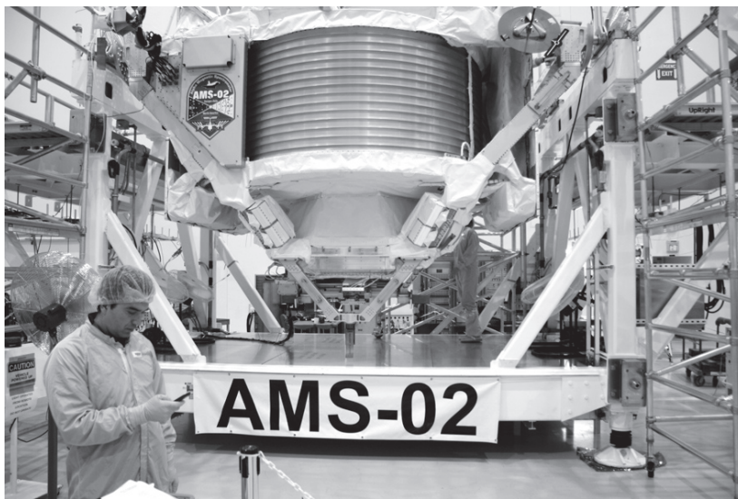
L'espectròmetre AMS-2.
