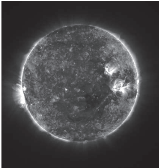
Imagen del Sol capturada por la sonda «Stereo» (NASA).
