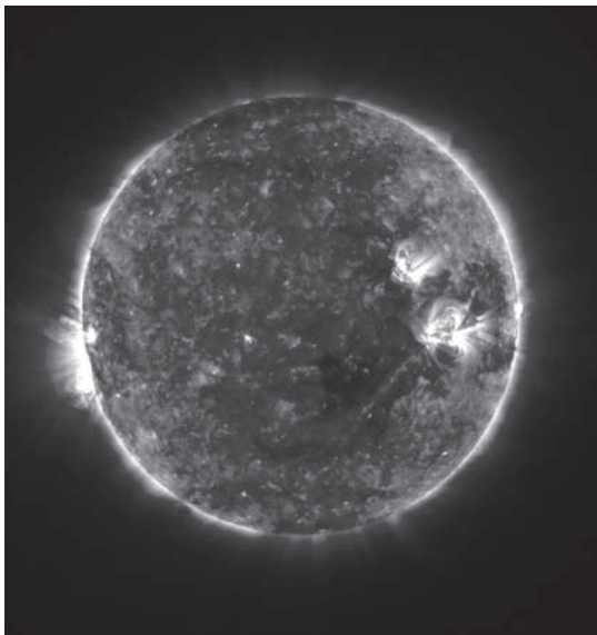
Imatge del Sol capturada per la sonda « Stereo » (NASA).
