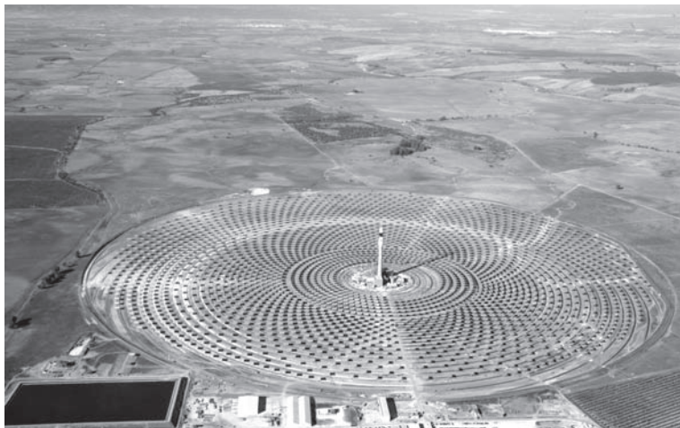
Helióstatos de la central solar termoeléctrica «Gemasolar», en Fuentes de Andalucía (Sevilla).
