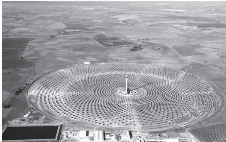
Heliòstats de la central solar termoelèctrica «Gemasolar», a Fuentes de Andalucía (Sevilla).
