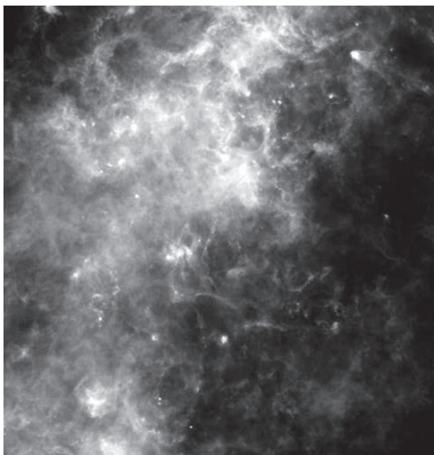
Nube cósmica.
