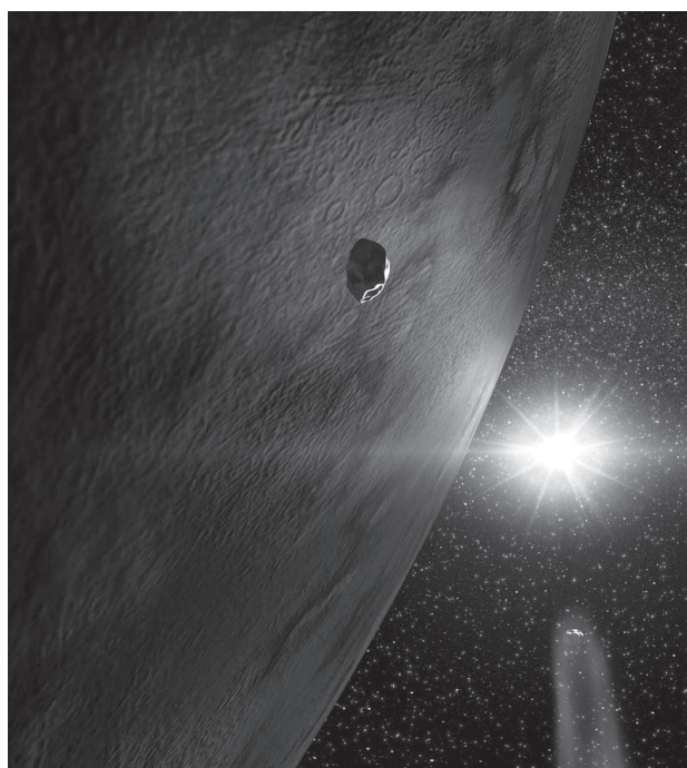
Recreación del asteroide 24 Themis y dos fragmentos desprendidos (uno de ellos con cola tipo cometa).
