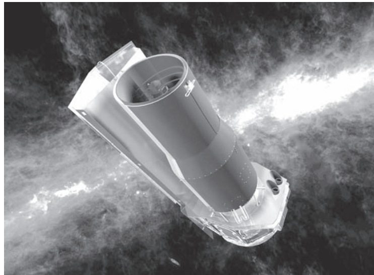
Telescopio «Spitzer».
