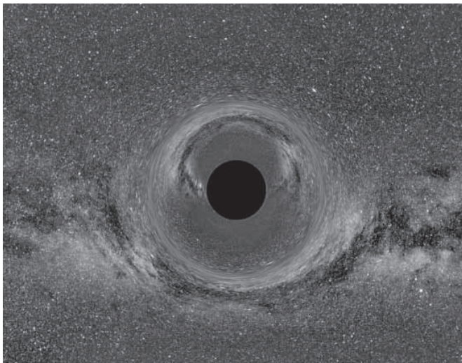
Representació d'un forat negre.
