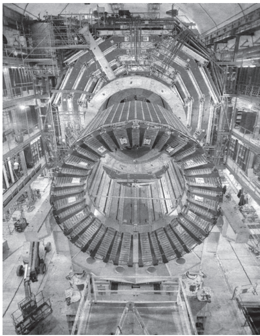
El Gran Col·lisionador d'Hadrons.
