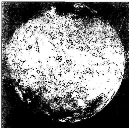
Un dels satèl·lits de Júpiter, Ío.
