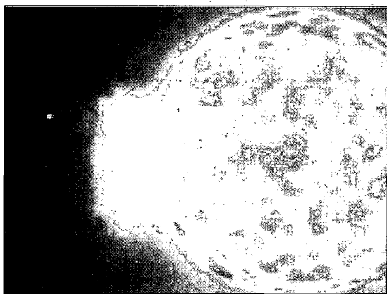
Simulació del procés d'impacte del planeta.
