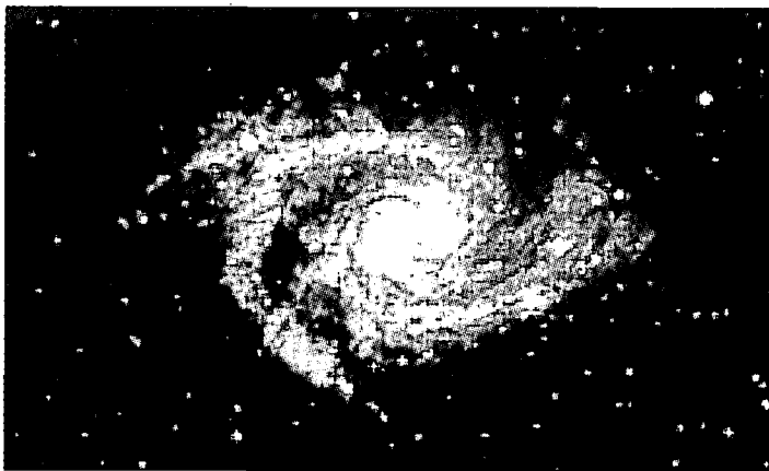
Galàxia espiral.
