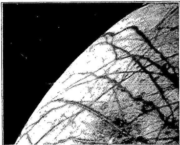
Impressionant vista del satèl·lit Europa solcat de ratlles fosques, va ser presa pel Voyager 2 .
