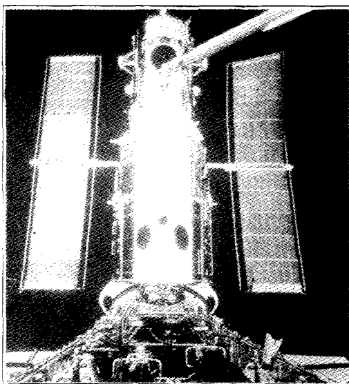
El telescopi «Hubble».
