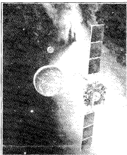
Imatge del telescopi «Chandra» creada per ordinador.
