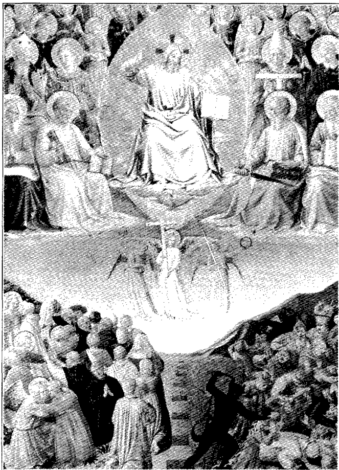
Detall del Tríptic del Judici Universal de Fa Angélico.
