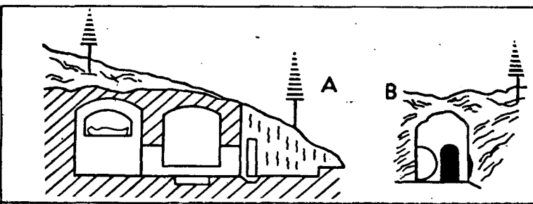
Model de tomba jueva excavada a la roca: A) Secció. B) Tanca.
